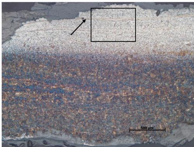
Figur 7. Fynd 95. Foto från mikroskopet på polerad och etsad yta. Samma utsnitt som i figur 4. I den övre ljusare delen ett lågkolhaltigt stål (mest ferrit). I den nedre mörkare delen stål med högre kolhalt (brunblå perlit). Långsmala, ljus bruna stråk längs med bildens långsida är vällfogar. Pilen visar analys P5 i vällfogen, med högt nickelnehåll.
