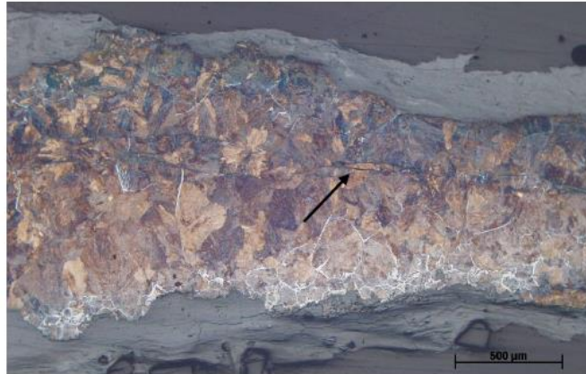
Figur 11. Fynd 103. Foto från mikroskopet på polerad och etsad yta. Metallen utgörs av stål med hög kolhalt (brunblå perlit). Mot den nedre ytterkanten ses större andel ferrit (ljusa kornkontakter), dvs. lägre kolhalt. Centralt ses vindlande, men långsträckta, mörka, slagginnestutningar som utgörs av en glasfas (pilen, jämför liknande i föregående figur).
