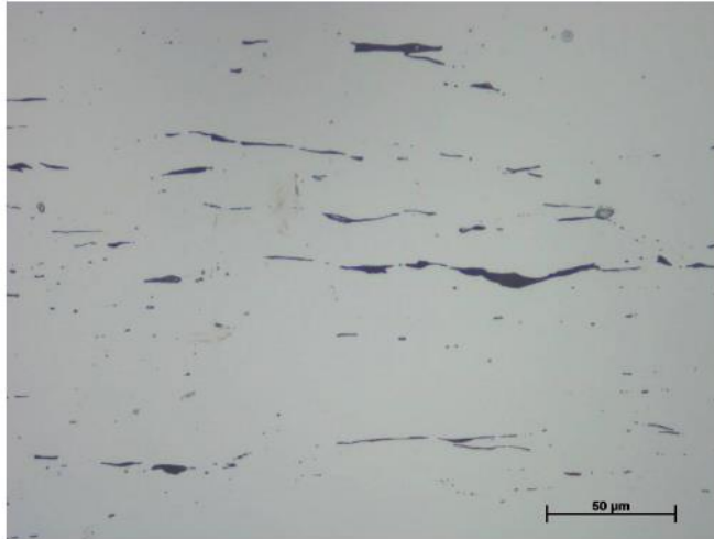
Figur 6. Fynd 95. Foto från mikroskopet på polerad yta; detalj från nedre delen i figur 4 på slagginneslutningar. Här utgörs de främst av en mörkt grå glasfas.
