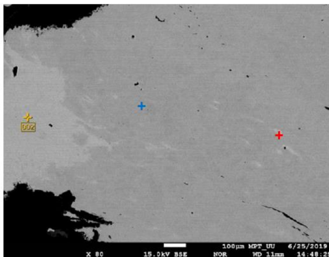
Figur 20. Fynd 131. Foto från elektronmikrosonden. Det blå plusset är analys i perlit (mörkare grå, analys P3) medan det gula (analys P4) är analys i ett ljusare grått område av samma typ som i de ljusare vällfogarna (röd, analys P5); de båda senare med högre nickel. De tunna svarta stråken i nedre högra hörnet är slagginneslutningar.
