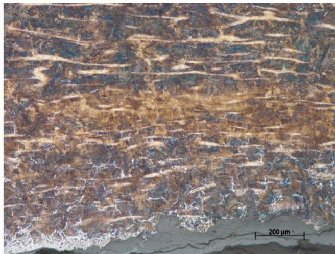
Figur 19. Fynd 131. Foto från mikroskopet på polerad och etsad yta. Stora delar utgörs av stål med hög kolhalt (brunblå perlit). Längst ned i bild, mot grå rostig ytterkant finns ett område med lägre kolhalt (där vita ytor är ferrit).
