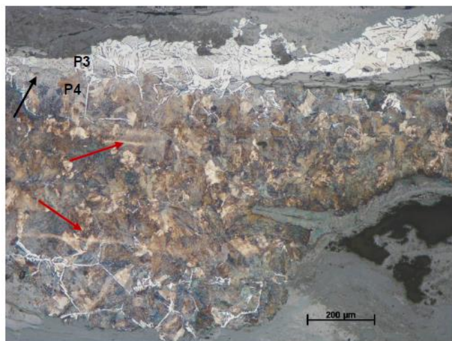
Figur 15. Fynd 104. Foto från mikroskopet på polerad och etsad yta från rutan i figur 13. I den övre, tunnare, ljusare delen ett lågkolhaltigt stål (mest ferrit). I den nedre mörkare delen stål med högre kolhalt (brunblå perlit). Långsmala, ljus bruna stråk (röda pilar) längs med bildens långsida är vällfogar. Slaggen från område 1 i föregående figur ses vid den svarta pilen. Omgivande grå ytor är rost. Analyserna P3 och P4 är markerade överst i bild.
