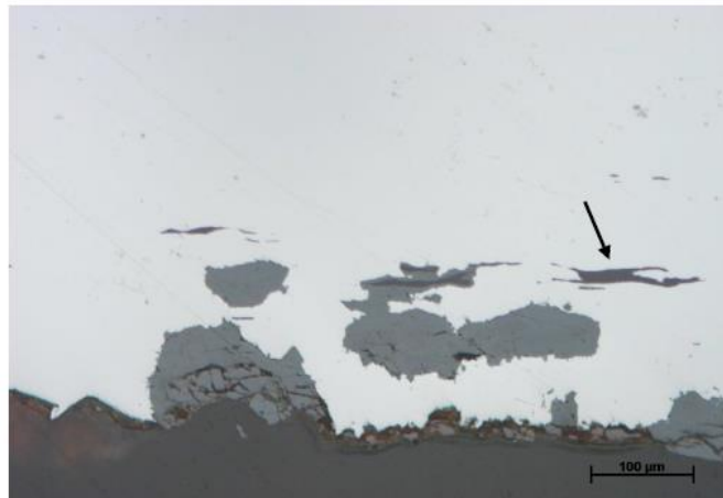
Figur 23. Fynd 144. Foto från mikroskopet på polerad yta; detalj från vänstra delen (rutan) i föregående figur på slagginslutningar. Dessa utgörs främst av en mörkt grå glasfas (exempel vid pilen). Något ljusare grå ytor är rost.
