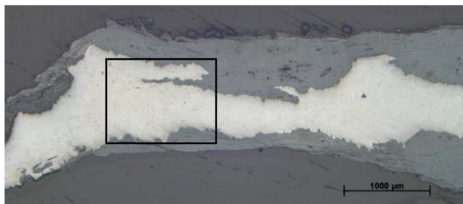
Figur 24. Fynd 144. Foto från mikroskopet på polerad och etsad yta. Samma utsnitt som figur 22. Metallen är ett i det närmast kolfritt järn. Ferrittexturen ses som (diffust) ljus bruna fält (se detalj från rutan i följande figur i högre förstoring).
