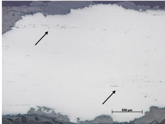
Figur 4. Fynd 95. Foto från mikroskopet på polerad yta. Hela provets tvärsnitt ses i bild; det ljusa metalliska järnet omges av grå rost på ömse sidor (överst och nederst). De tunna, långsträckta grå "fläckarna" är slagginneslutningar (pilarna); detalj i följande figurer.
