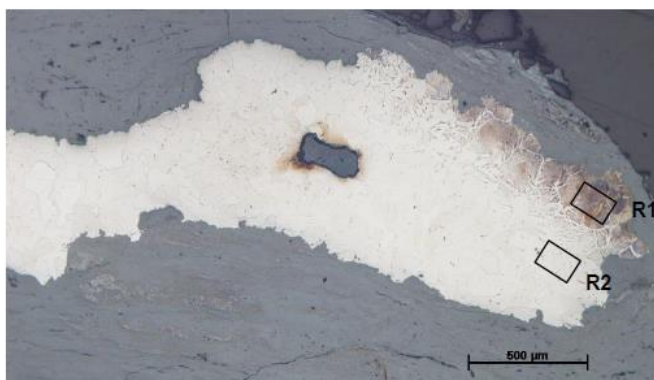
Figur 27. Fynd 144. Foto från mikroskopet på polerad och etsad yta. Detalj från kanten av provet där kolhalten lokalt är högre (brunblå perlit). Rutorna R1 och R2 är analyserade kemiskt.
