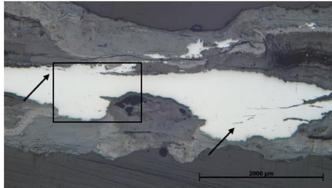
Figur 13. Fynd 104. Foto från mikroskopet på polerad yta. Centralt ses det ljusa metalliska järnet som är omgivet av tämligen mycket rost (flera grå nyanser). Några stråk av långsträckta slagginneslutningar kan också ses (pilarna). Detalj på etsat prov från den markerade rutan visas i figur 15.
