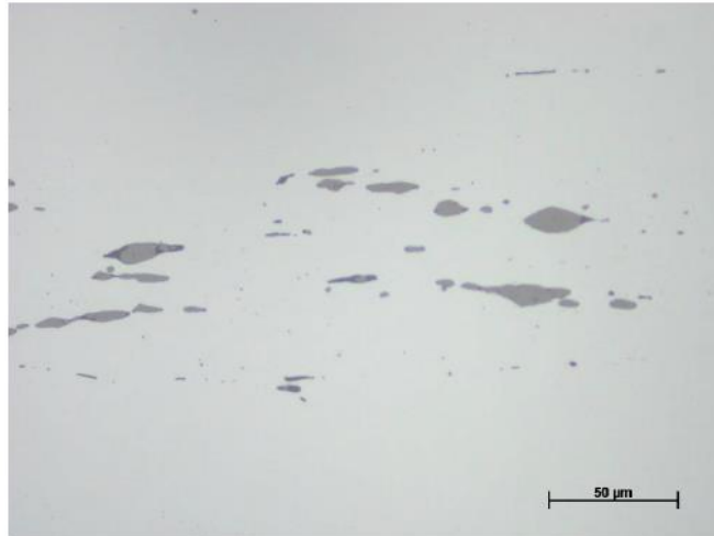
Figur 5. Fynd 95. Foto från mikroskopet på polerad yta; detalj från övre delen i föregående figur på slagginneslutningar. Dessa utgörs främst av wüstit (grå). I någon ses små mörkare ytor som är en glasfas (jämför nästa figur).
