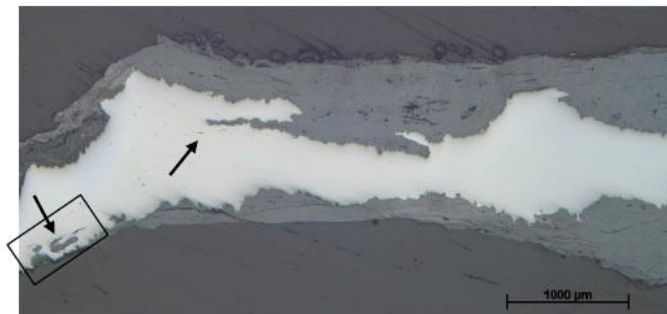
Figur 22. Fynd 144. Foto från mikroskopet på polerad yta. Centralt ses det ljusa metalliska järnet som är omgivet av tämligen mycket rost (flera grå nyanser). Några stråk av långsträckt slagginslutningar kan också anas vid pilarna (se följande figur).
