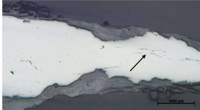
Figur 10. Fynd 103. Foto från mikroskopet på polerad yta. Centralt i det ljusa metalliska järnet ses tunna, något vindlande, men långsträckta, mörka, slagginnestutningar som utgörs av en glasfas. Metallen omges av grå rost.
