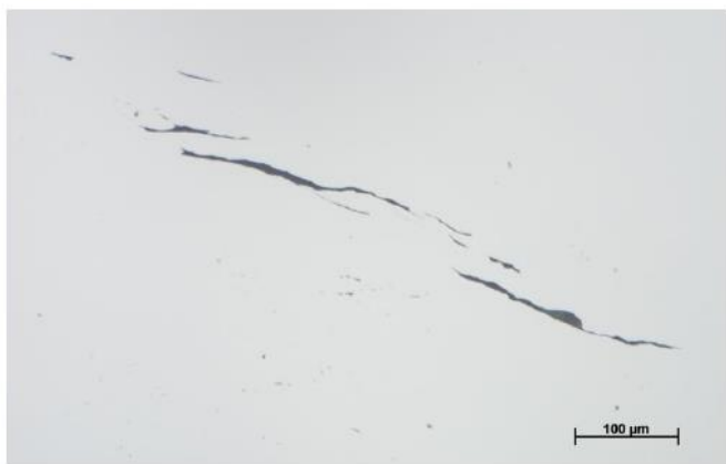
Figur 18. Fynd 131. Foto från mikroskopet på polerad yta; detalj från övre delen i föregående figur på slagginneslutningar som utgörs av en glasfas.
