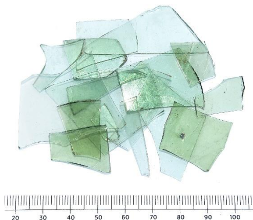
Figur 93. Fönsterglas (Fnr 16).
