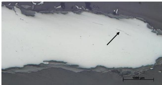
Figur 17. Fynd 131. Foto från mikroskopet på polerad yta. Centralt ses det ljusa metalliska järnet omgivet av en tunn hinna av rost (flera grå nyanser). Några enstaka stråk av långsträckt slagginneslutningar kan också ses (pilen).
