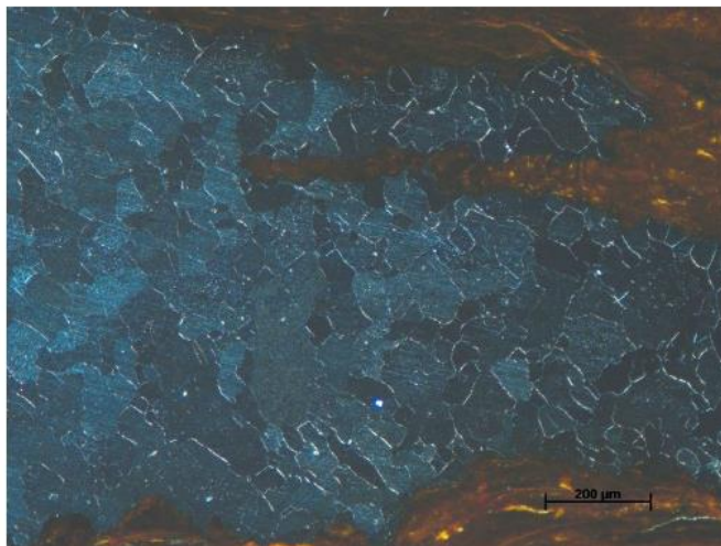
Figur 26. Fynd 144. Foto från mikroskopet på polerad och etsad yta. Samma utsnitt som föregående figur, men en inställning i mikroskopet där ferritkornen är mörkt grå och kontakterna lyser ljusa och tydligt visar kornform och storlek. Omgivande rost är brunröd.
