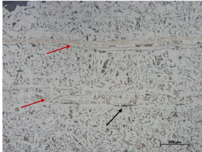
Figur 8. Fynd 95. Foto från mikroskopet på polerad och etsad yta. Detalj från rutan i föregående figur. Ljusa ytor är ferrit, bruna är perlit. Ljust bruna stråk (röd pil) markerar vällfogar; i den nedre också med långsmala grå slagginneslutningar (svart pil).
