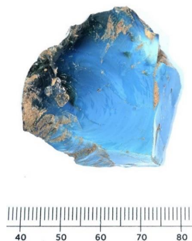
Figur 102. Masugnsslagg (Fnr 35).
