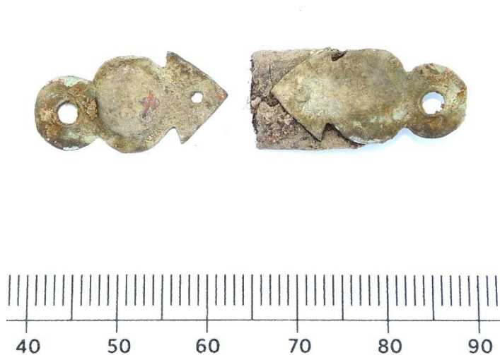
Figur 123. Bokspännen (Fnr 14).
