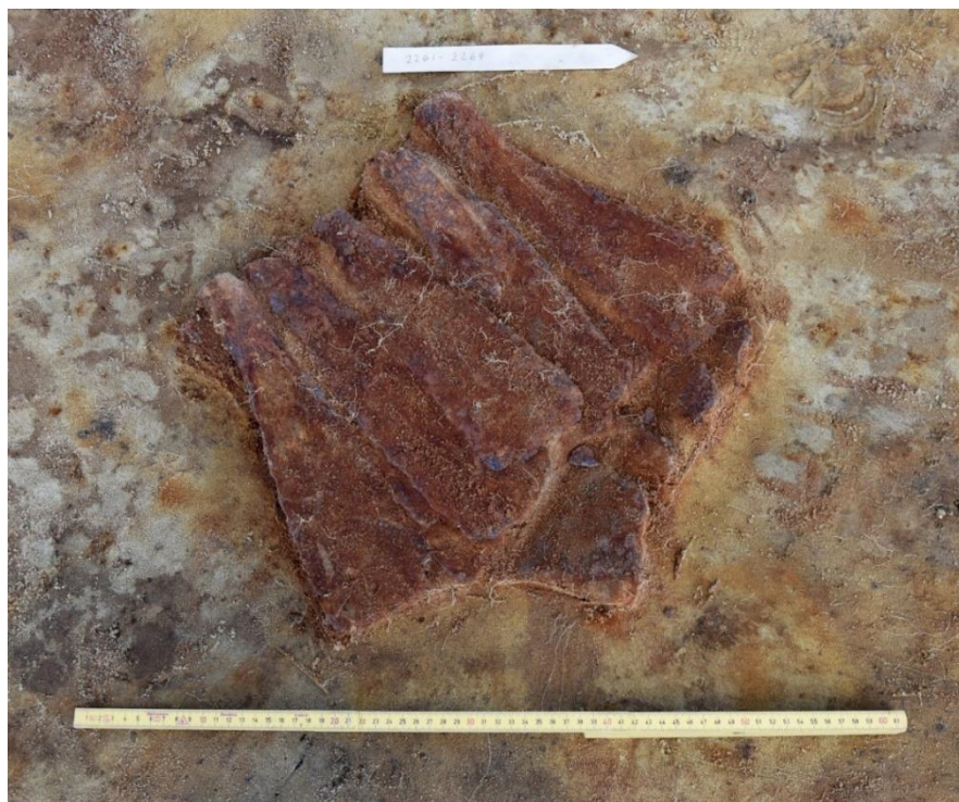
Figur 40. Ämnesjärnsdepå 2 (2261-2269).
