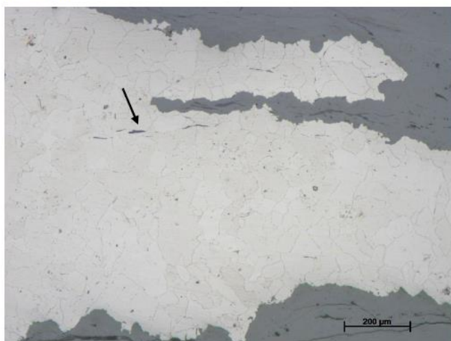
Figur 25. Fynd 144. Foto från mikroskopet på polerad och etsad yta. Detalj från rutan i föregående figur. De oregelbundet formade, ljusa ferritkornen urskiljs med hjälp av tunna svarta kontakter (se även följande figur). Vid pilen ses tunna mörkt grå slagginslutningar. Omgivande rost är grå.
