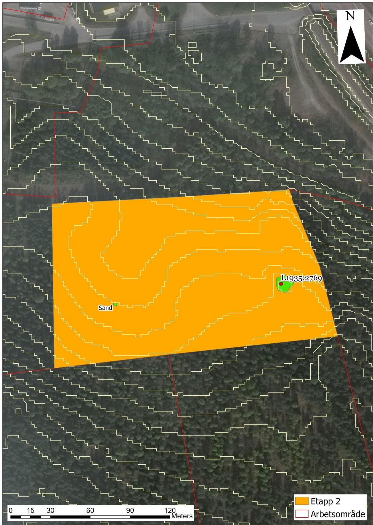
Figur 16. Utredningsområdet i område 14 omkring röset L1935:2769 och ett flackare område med sandig jord. Strandlinjer visar det flackare området.
