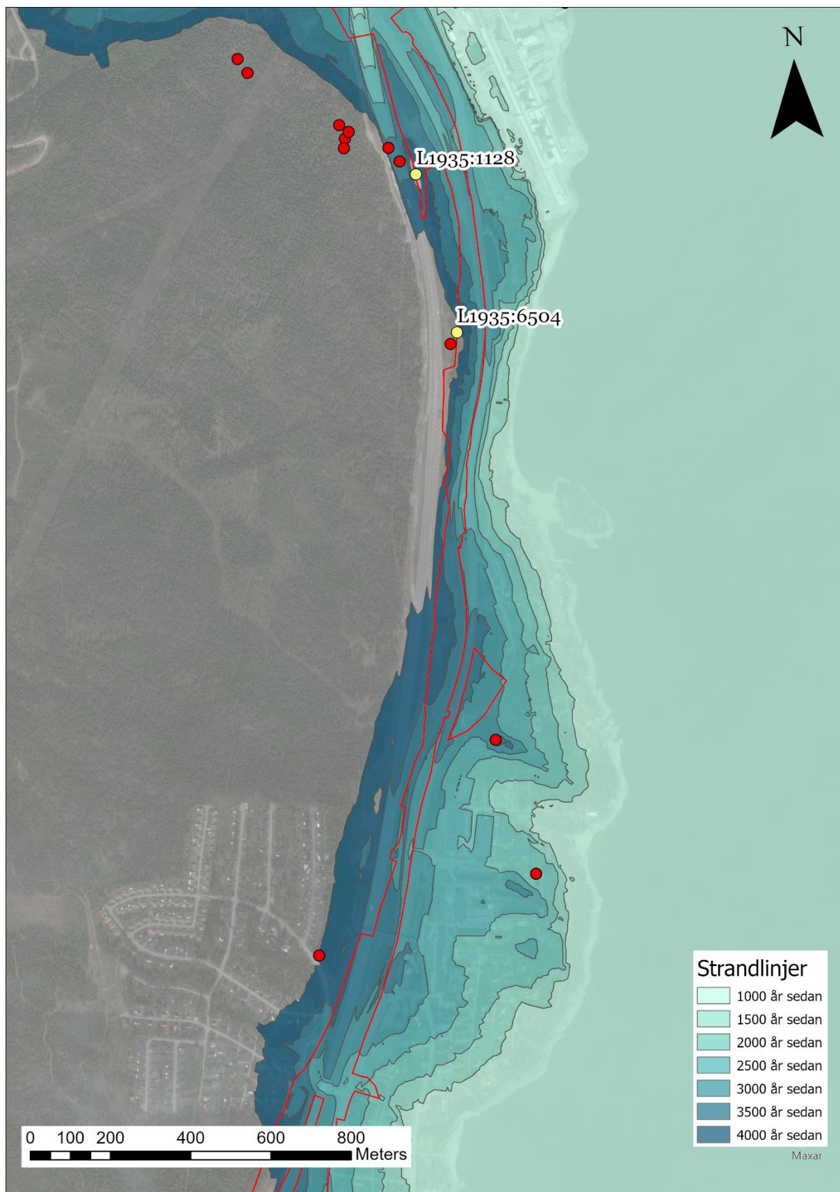
Figur 9. Strandlinjer över arbetsområdet från 1000–4000 år sedan.
