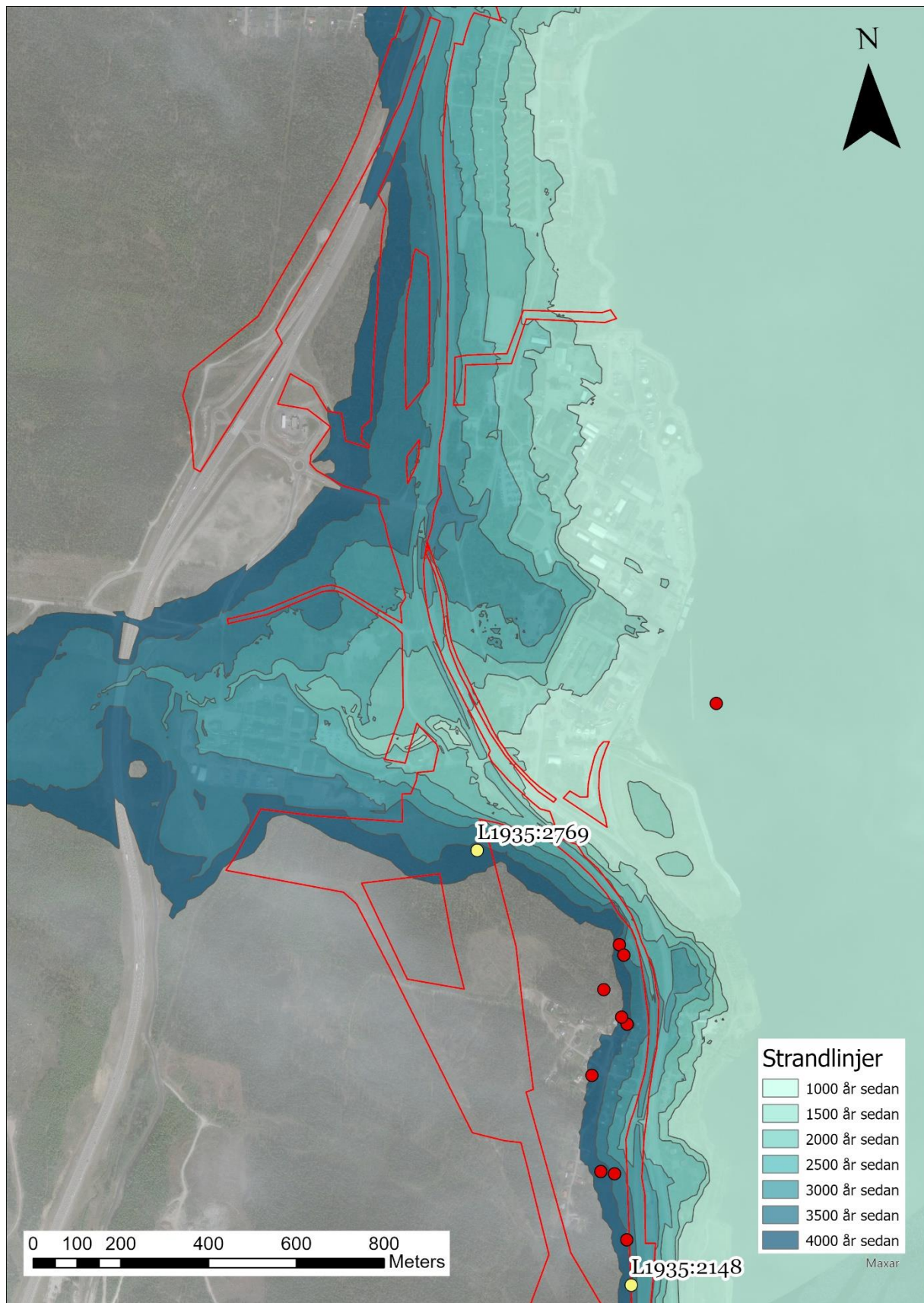
Figur 10. Strandlinjer över arbetsområdet från 1000–4000 år sedan.
