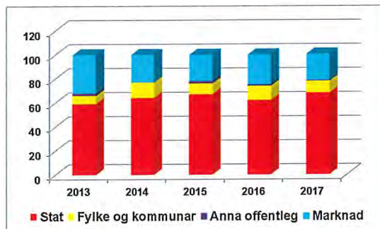
Figur 3. Inntektsprofil 2013–2017 Prosent
