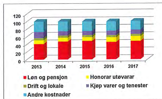
Figur 18. Kostnadsprofil 2013–2017 Prosent
