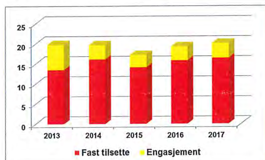
Figur 4. Betalte årsverk 2013–2017
