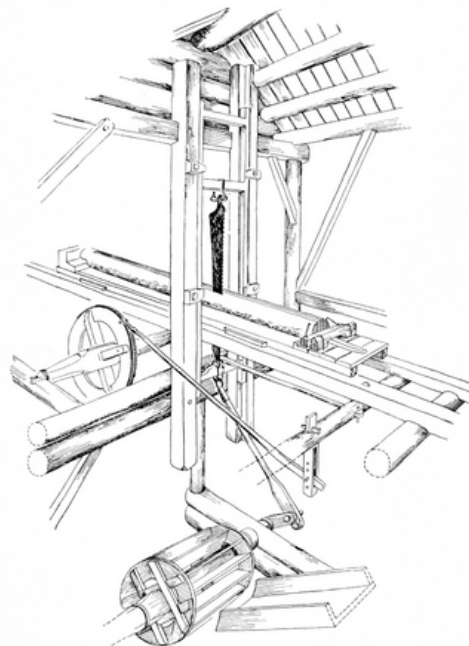
Skisse av de sentrale delene av en oppgangssag.
