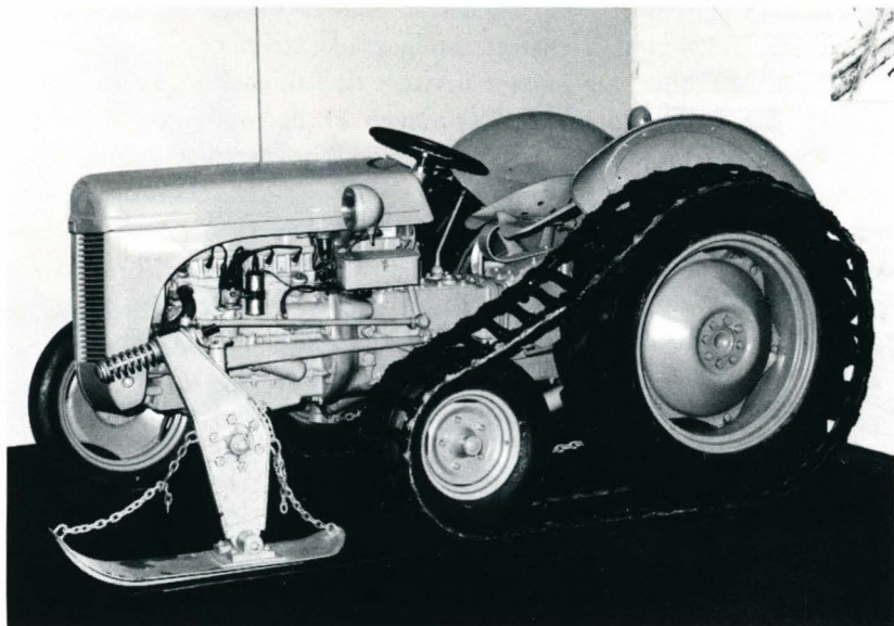
«Gråtass», museets Ferguson traktor med ski og halvbelter. Traktoren er en gave fra Eikmaskin, ski og halvbelter er gitt av Norsk Institutt for Skogforskning.
