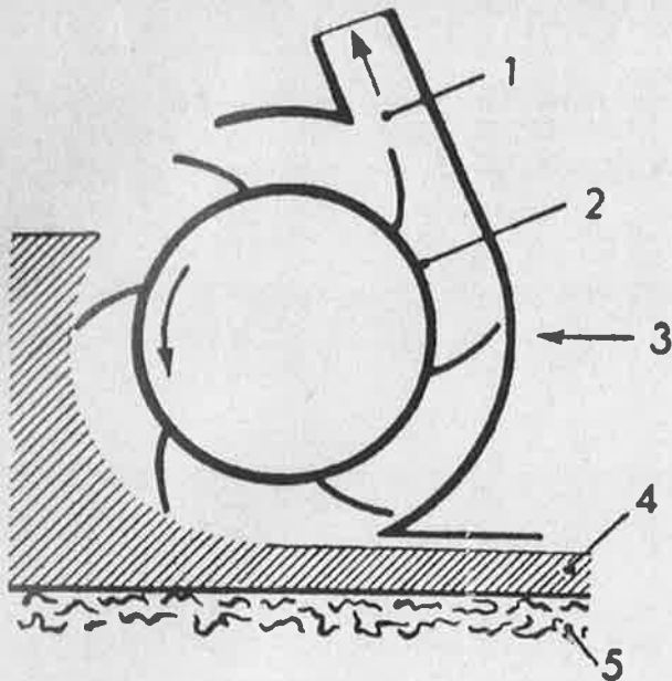
Fig. 4. Skjematisk snitt gjennom snøfreseren.
