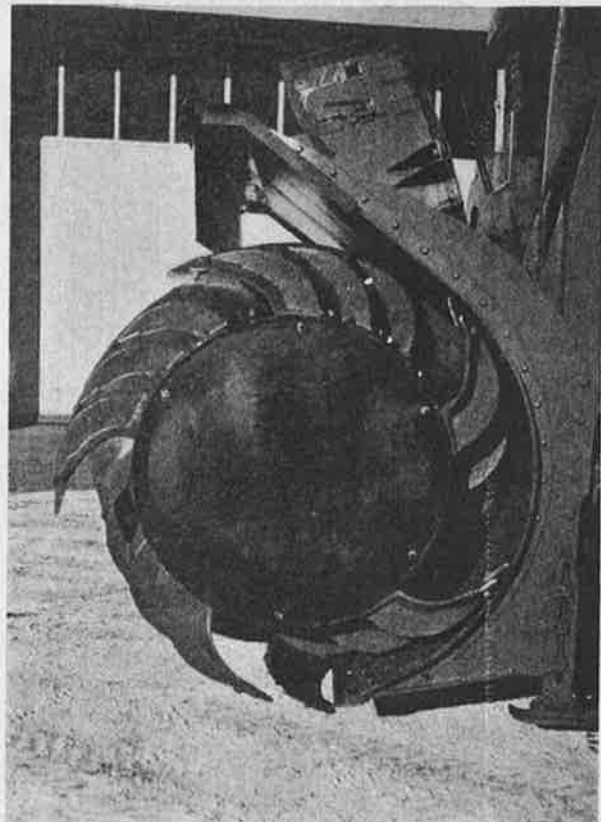
Fig. 5. Peters snøfreser. Fresevalsen sett fra siden.
